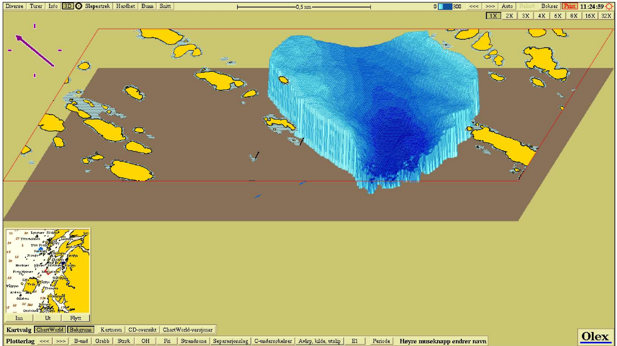
Figur 3.2. Eksempel på 3D visning av oppmålt batymetri.
